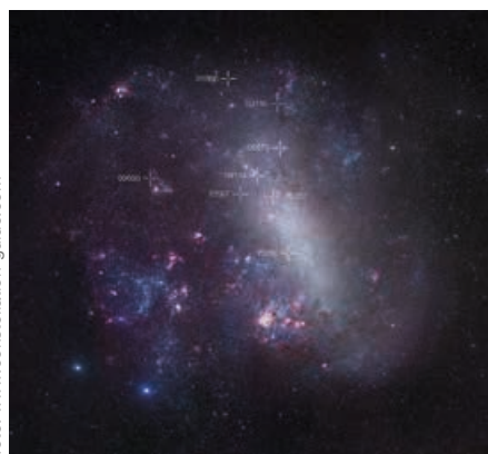
Velký Magellanův oblak, částečně se nacházející v souhvězdí Mensa
