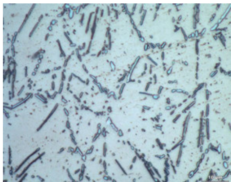
Slitina niklu – letecký motor
